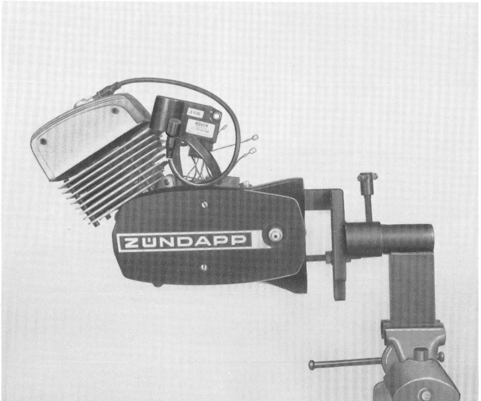
Motor mit Super-Therm-Zylinder in der Haltevorrichtung SK-A 314
