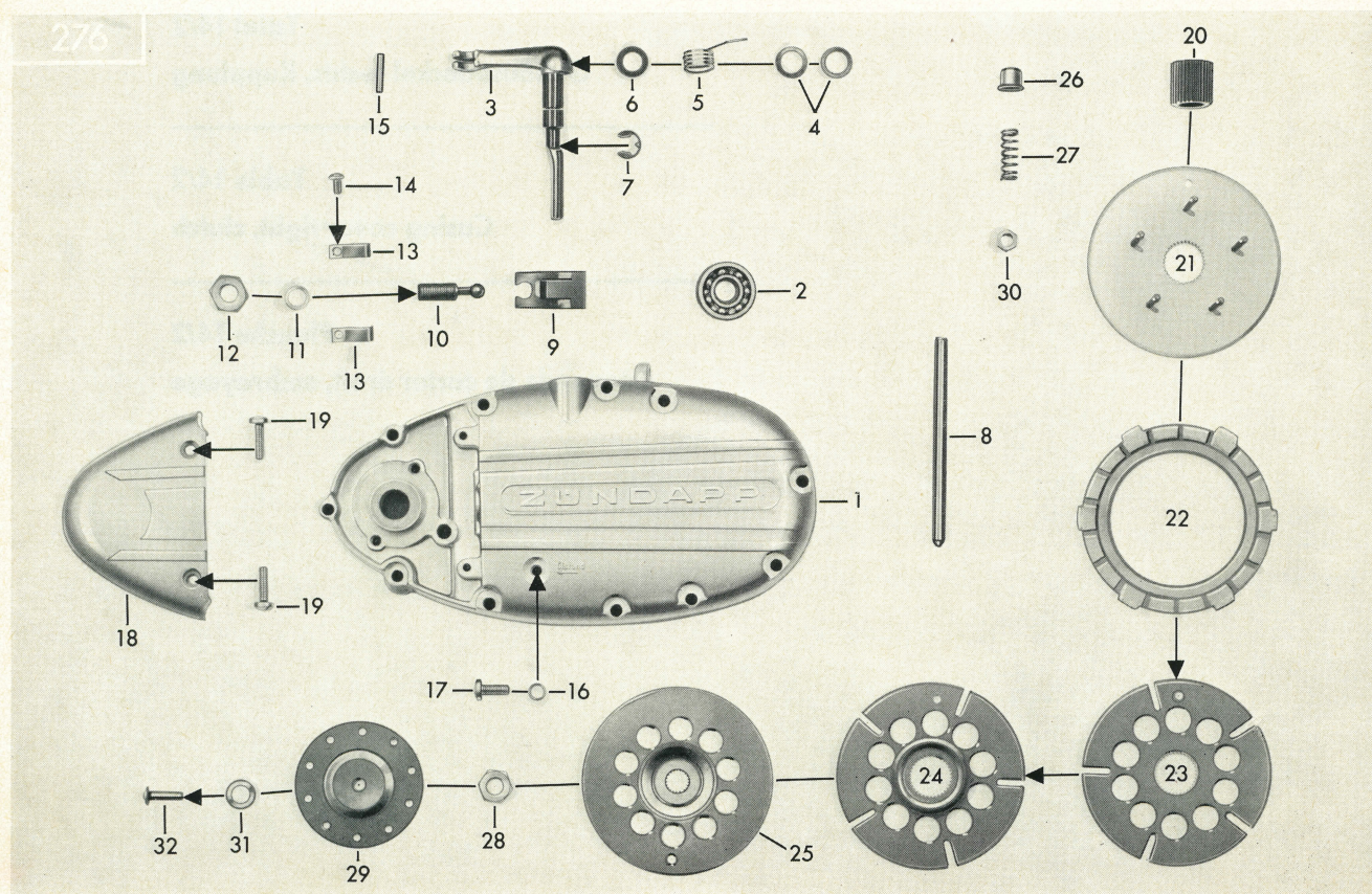
Tafel 14/2 Gehäusedeckel rechts, Kupplung Table 14/2 Casing cover right, clutch Planche 14/2 Couvercle de carter droit, embrayage
