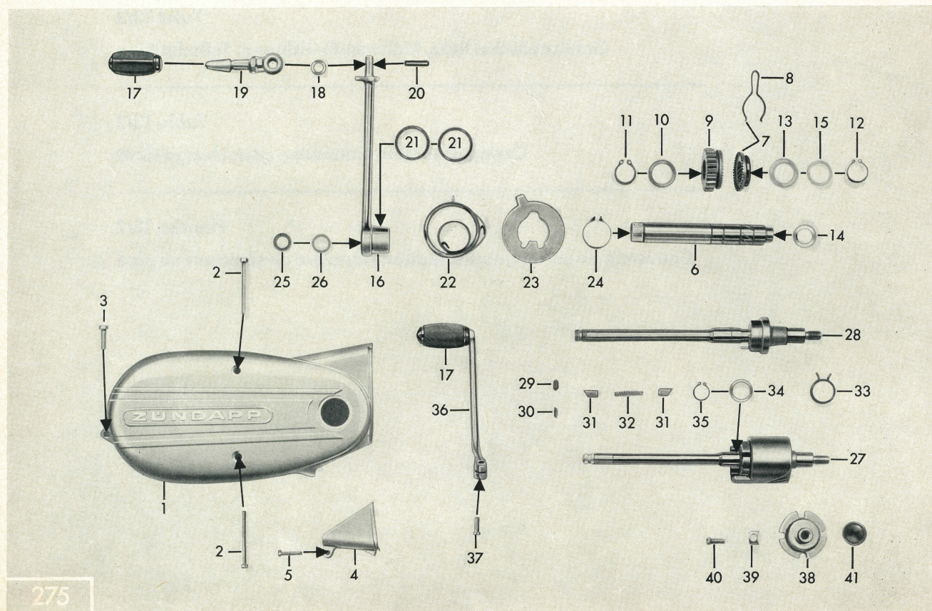
Tafel 13/2 Gehäusedeckel links, Kickstart-Einrichtung, Fußschaltung Table 13/2 Casing cover left, kickstarter, gear change shaft Planche 13/2 Couvercle de carter gauche, kickstarter, arbre de sélecteur au pied
