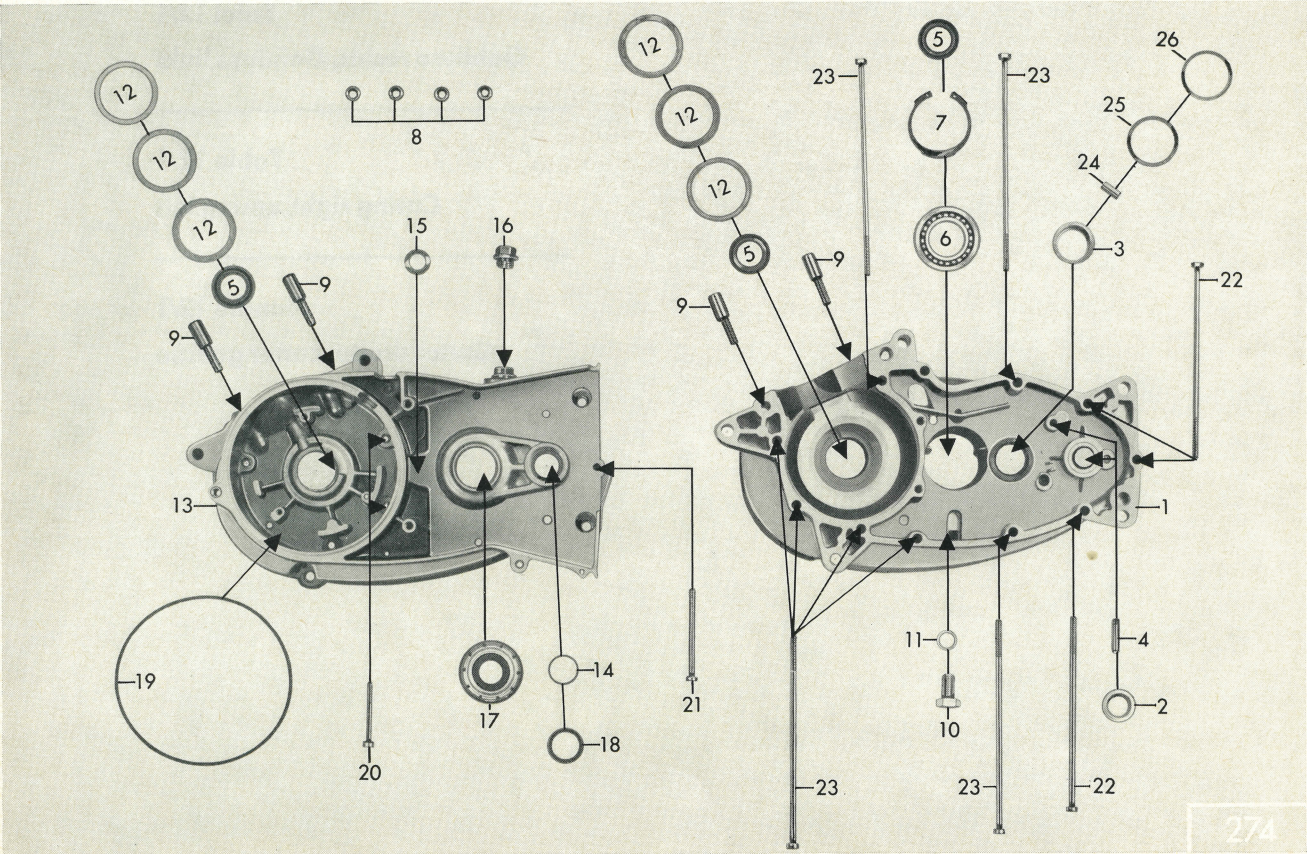
Tafel 12/1 Gehäuse rechts, Gehäuse links Table 12/1 Casing right, casing left Planche 12/1 Carter droite, carter gauche
