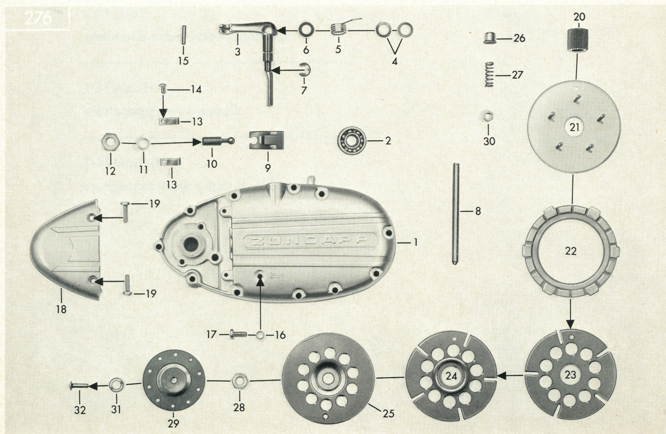
Tafel 14/1 Gehäusedeckel rechts, Kupplung Table 14/1 Casing cover right, clutch Planche 14/1 Couvercle de carter droit, embrayage
