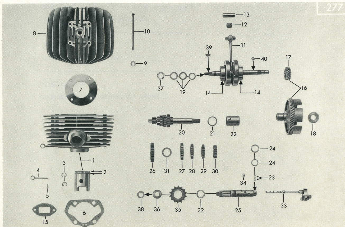
Tafel 15/2 Zylinder, Kurbelwelle, Getriebe Table 15/2 Cylinder, crankshaft, gearbox Planche 15/2 Cylindre, vilebrequin, boîte de vitesses
