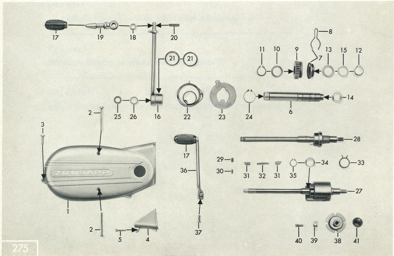
Tafel 13/1 Gehäusedeckel links, Kickstart-Einrichtung, Fußschaltung Table 13/1 Casing cover left, kickstarter, gear change shaft Planche 13/1 Couvercle de carter gauche, kickstarter, arbre de sélecteur au pied
