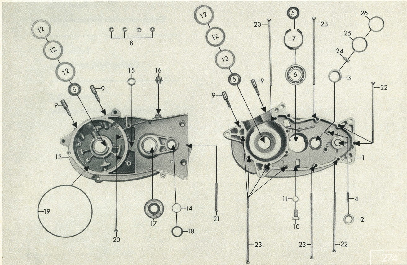
Tafel 12/2 Gehäuse rechts, Gehäuse links Table 12/2 Casing right, casing left Planche 12/2 Carter droite, carter gauche
